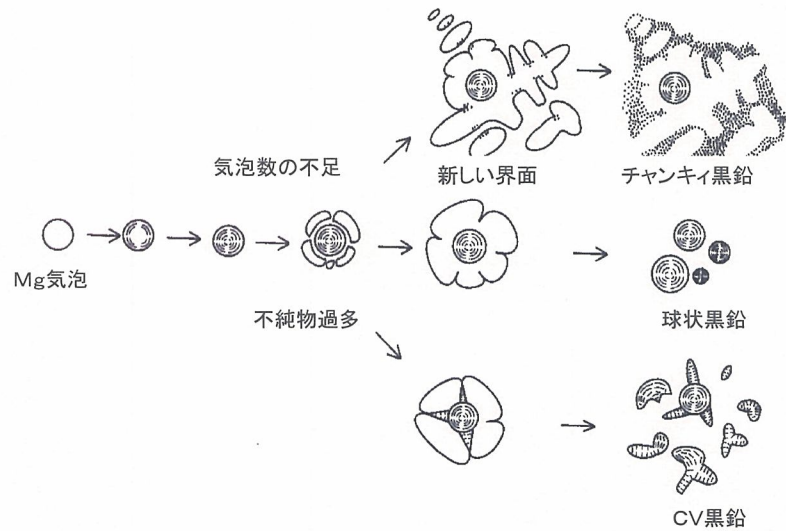
イラスト図. 黒鉛の球状及び退化メカニズム
