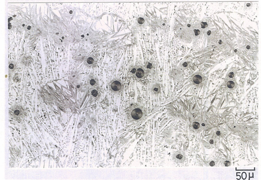
凝固途中で水冷したマイクロ組織; 3%ナイトル腐食
